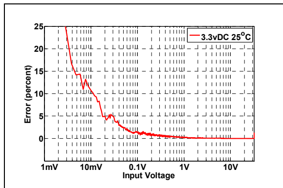
FIGURE 2-7: V_{BUS} Error vs. V_{BUS} Input Voltage.
