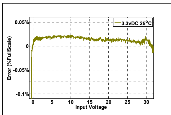
FIGURE 2-9: V_{BUS} Error vs. V_{BUS} Input Voltage.
