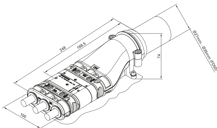
RobiFix-S35-ZEM
