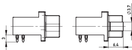
Mutter / nut
