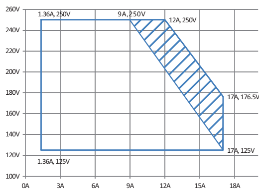
◎ CSP-3000-250
