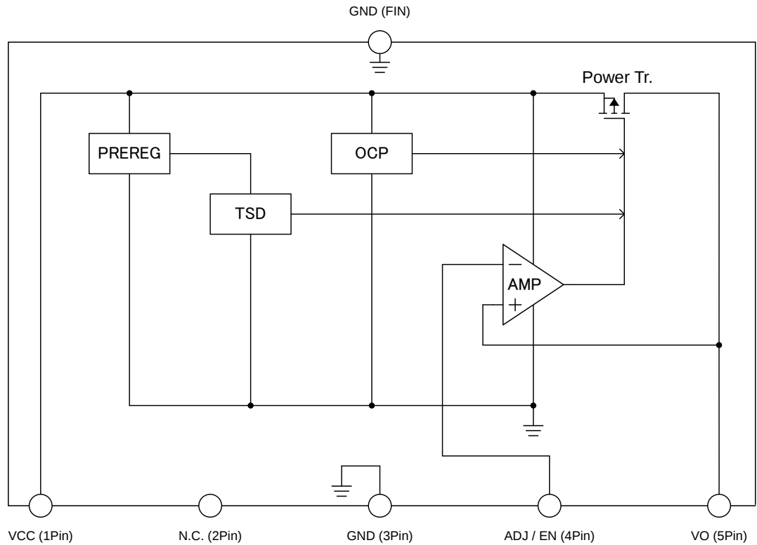
TO252-J5 / TO263-5
