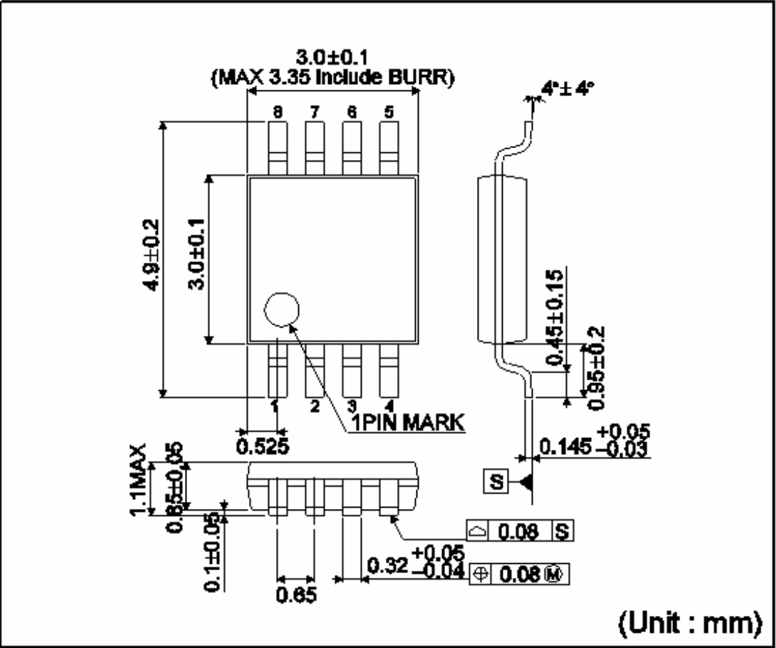
TSSOP-B8J
